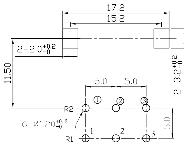
安裝孔位置圖 Mounting Hole
