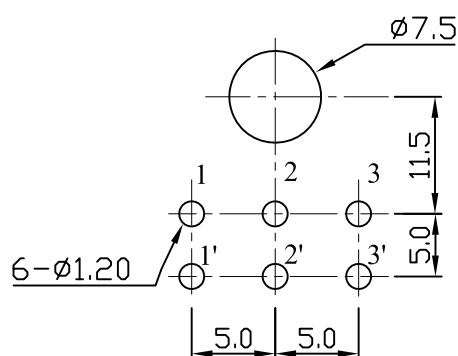
安裝孔位置圖 Mounting Hole
