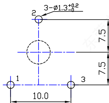
安裝孔位置圖 Mounting Hole
